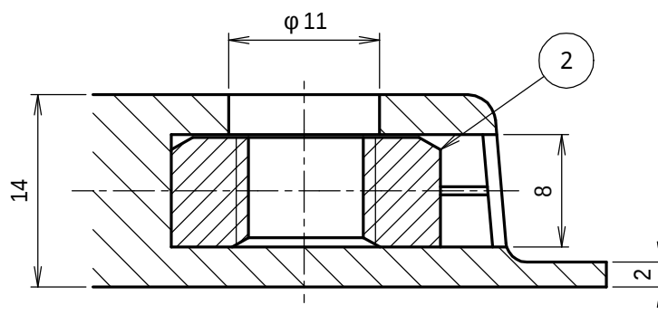
A-A断面図 (2/1)
